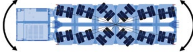
2. Karussell-Lenkung
