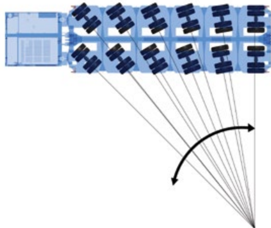
4. Vorderachslenkung
