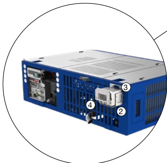
② FUNKEMPFÄNGER AM »ADDRONIC« HOST
